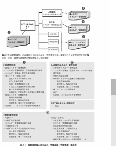
図-11 事業者組織とエネルギー管理規程 (管理標準) 構成例
